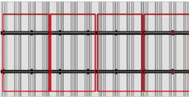
Figure 1 – Vue globale du procédé SPEEDRAIL SPEEDCLIP avec modules photovoltaïques posés en mode portrait
